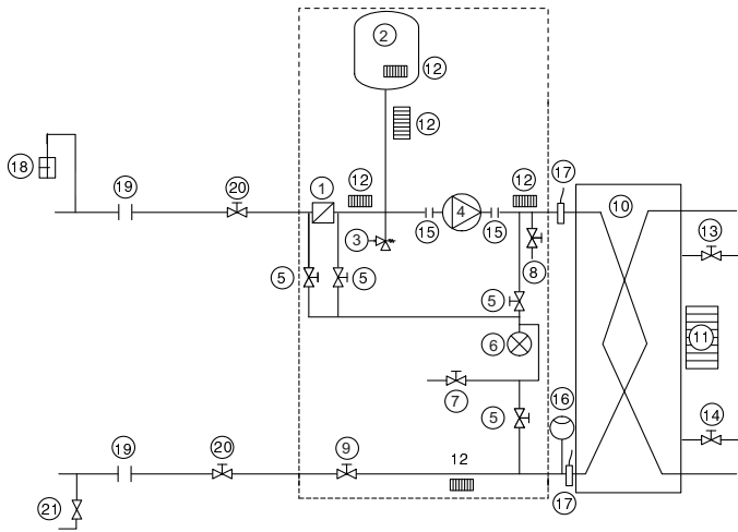
Principeschema van een watercircuit
